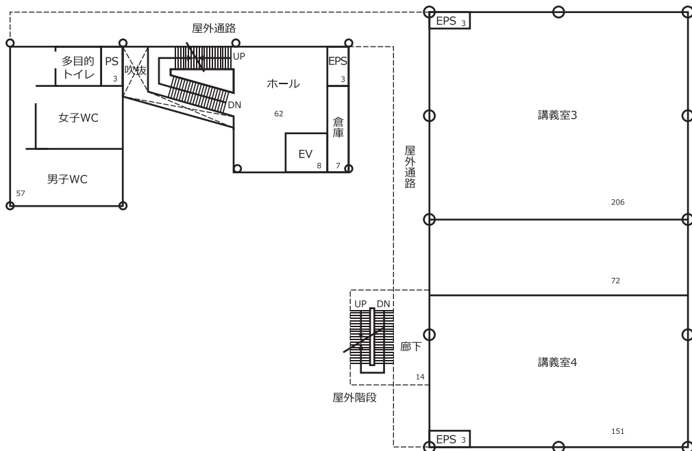
3階 599m 2
