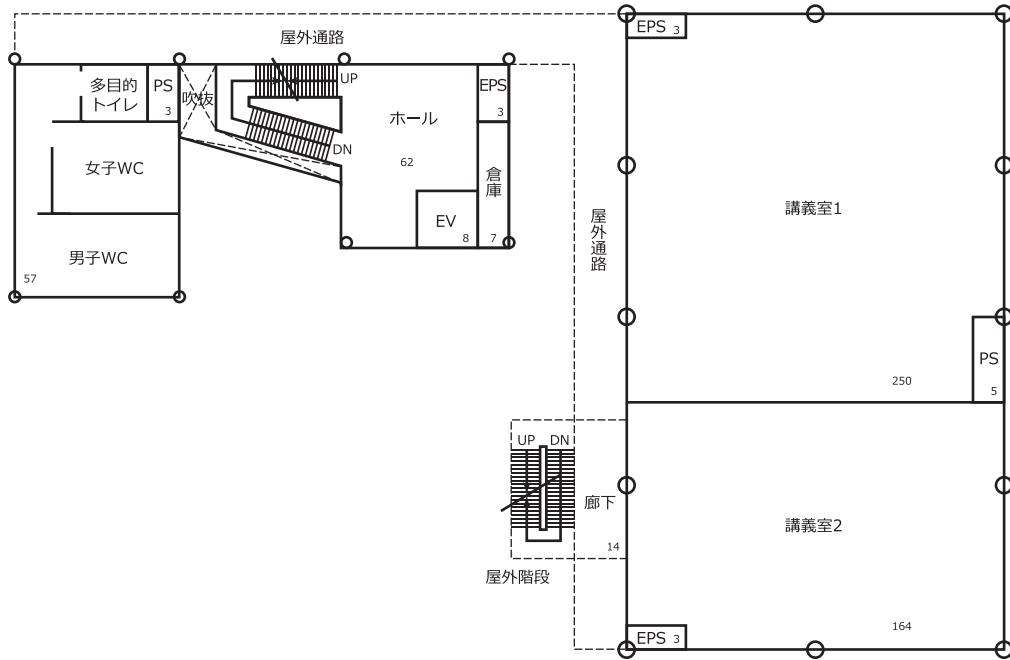
2階 599m 2
