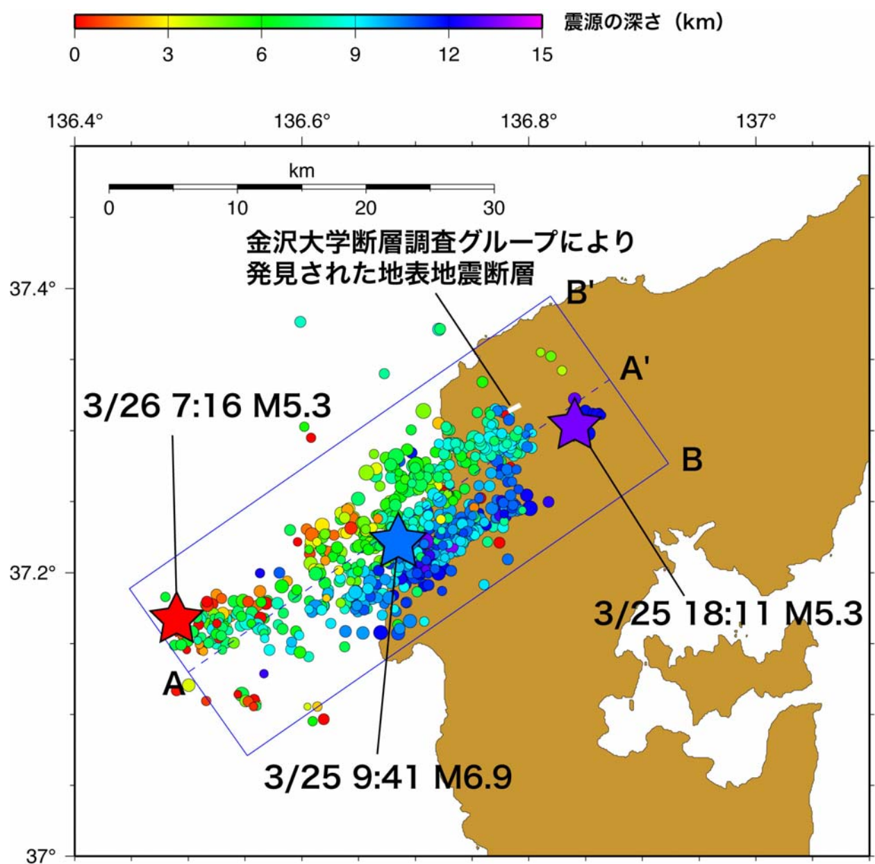
平成19年能登半島地震 余震分布 (3月25日~28日) 気象庁一元化震源データによる
