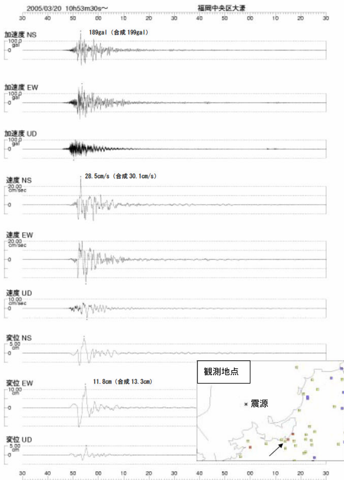
図 - 3 強震波形(気象庁) (福岡中央区大濠：震度 5 強、計測震度 5.1)
