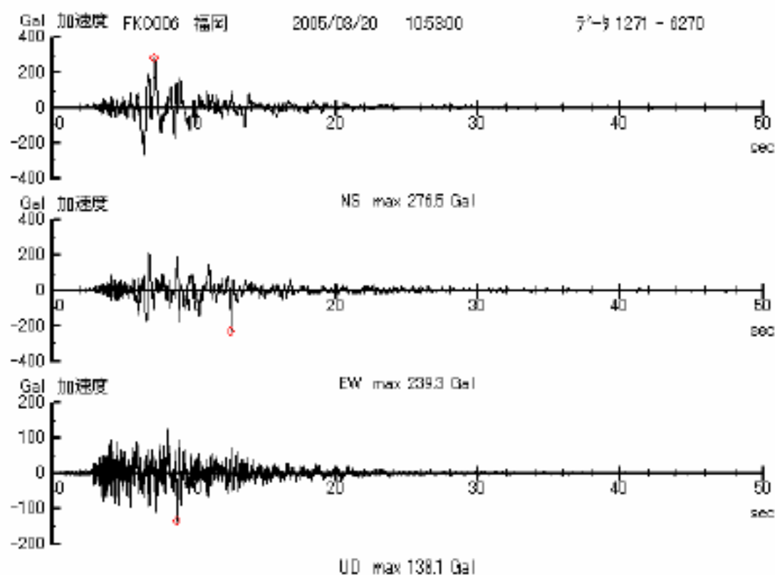
図 - 2 K-NET 福岡(FK0006)の観測記録(加速度時刻歴波形)
