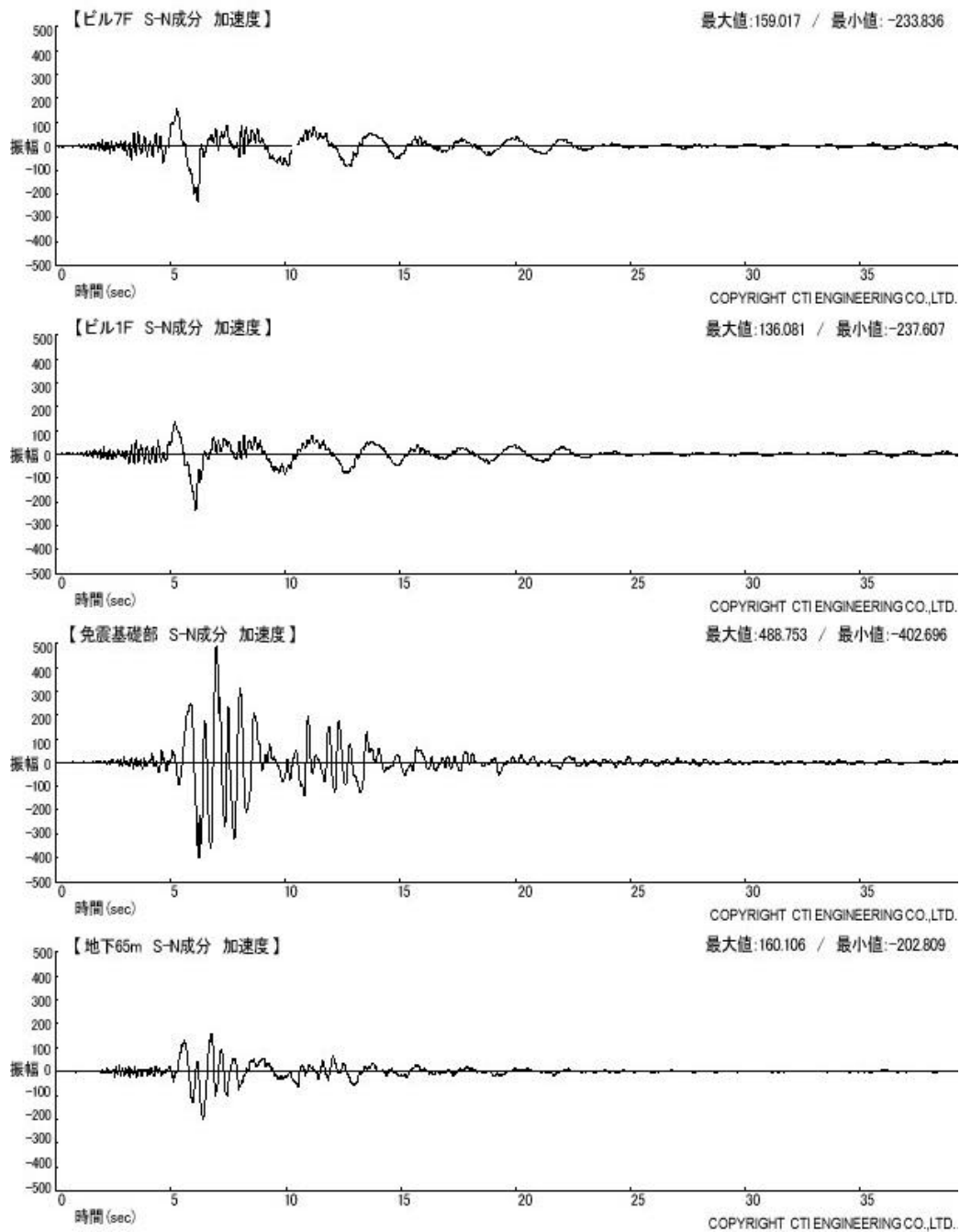
図 - 4 本震の加速度波形一覧表(CTI 福岡ビル)
