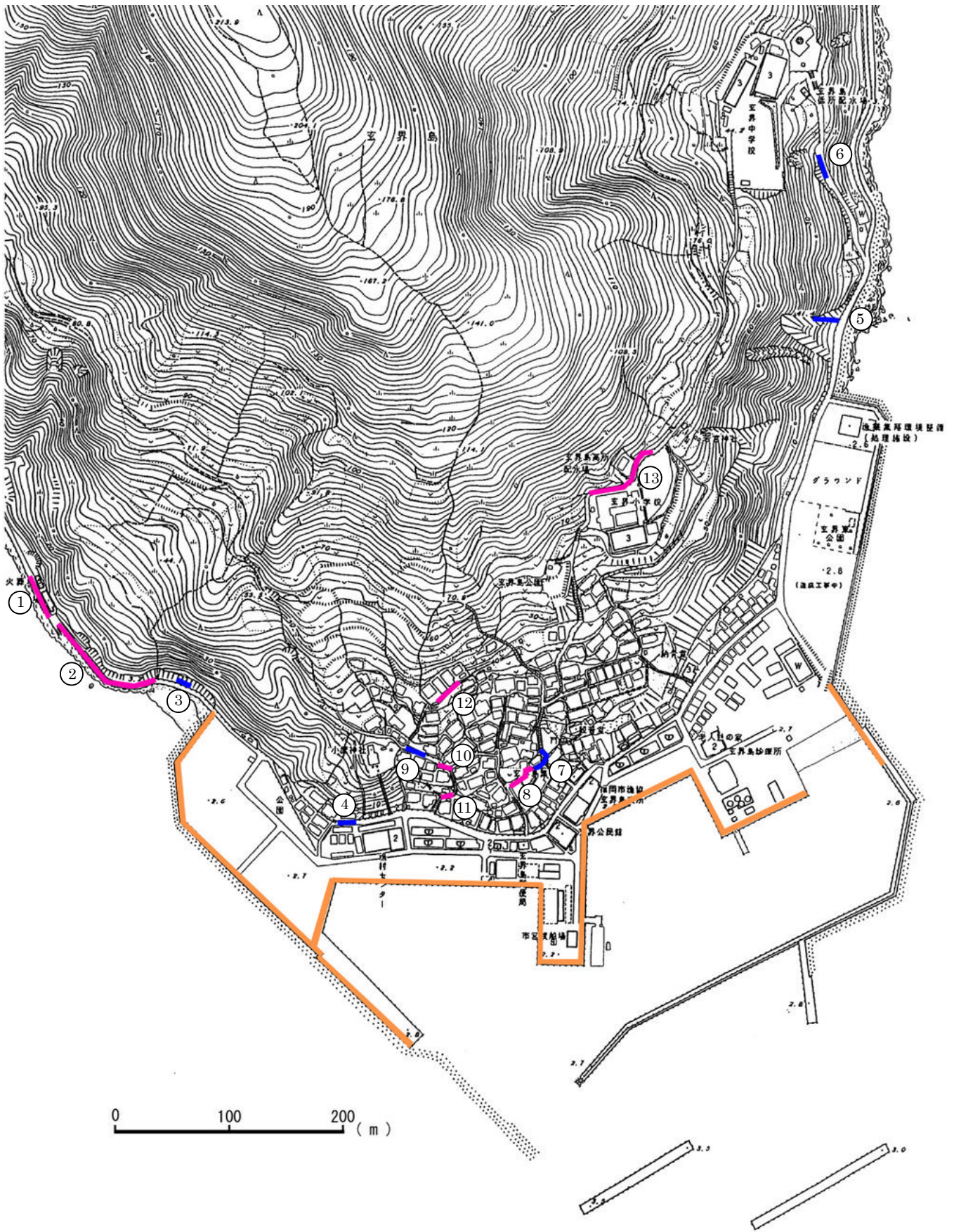
図 3.2.1 玄界島道路・漁港災害状況
