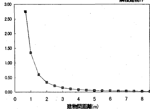
図 13 建物間距離と伝播係数
