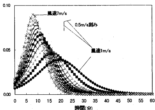
図 10 風速の違いに対する延焼力の変化
