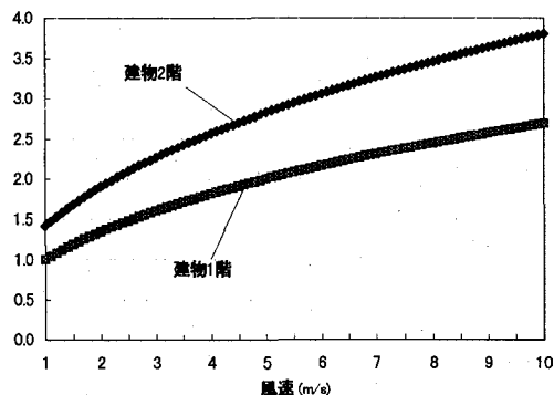
図 11 風速と伝播係数の関係
