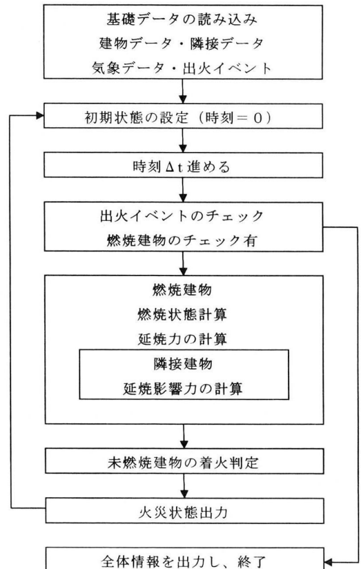
図 6 延焼シミュレーションフロー図
