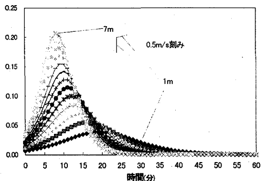
図 12 風速の違いに対する延焼影響量 (延焼力×伝播係数) の変化
