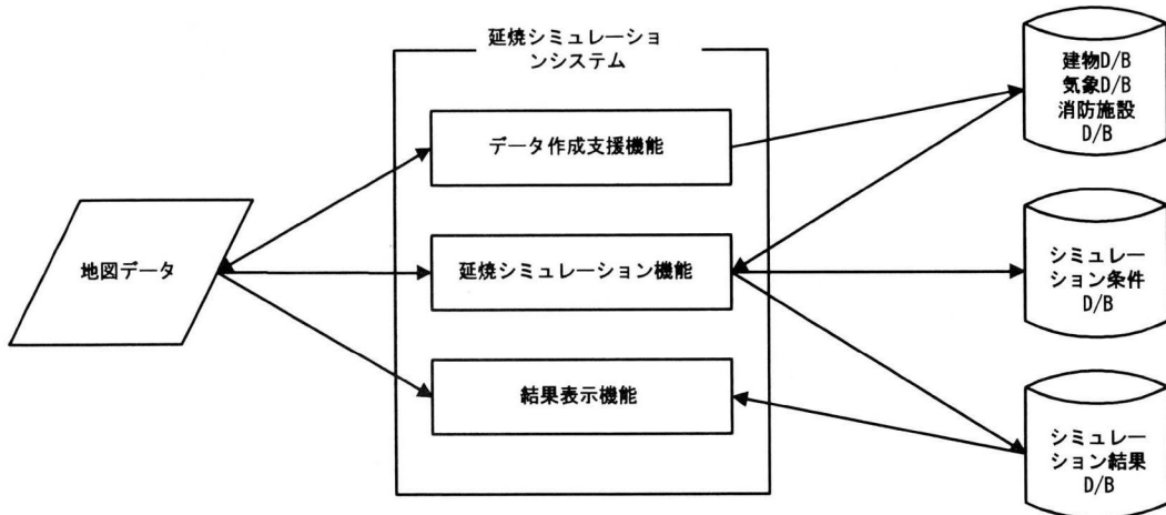
図2 延焼シミュレーションシステムの概要
