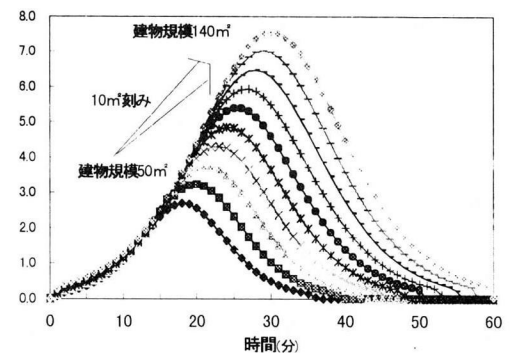
図 9 建物規模の変化に対する延焼力の変化
