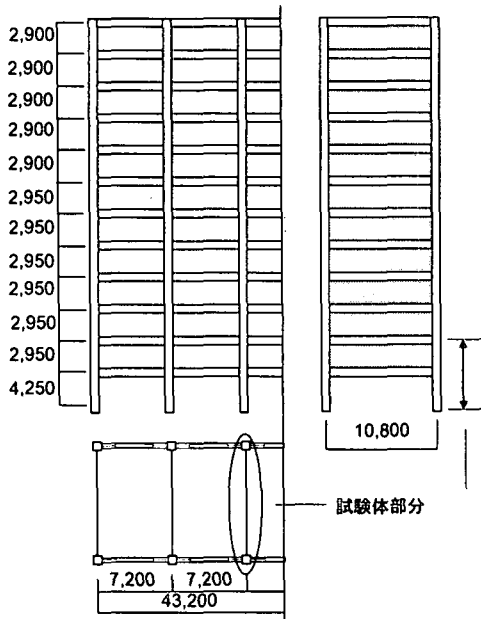
図-1 プロタイプ建築物概要 (単位: mm)
