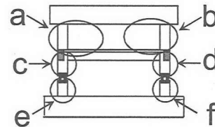
写真-1 最終破壊状況
