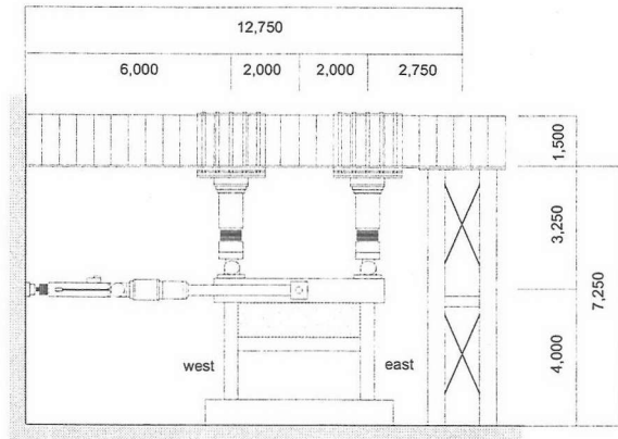
図-5 加力装置 (単位: mm)
