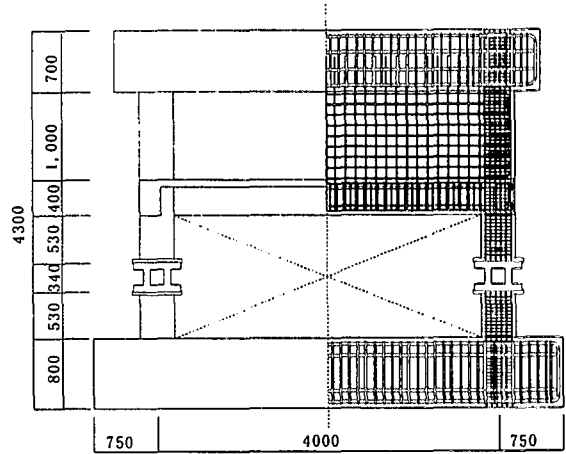
図-3 試験体の形状及び配筋 (単位: mm)
