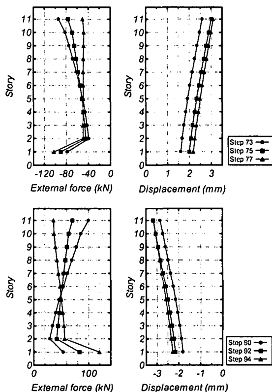
図-8 外力分布および変形分布
