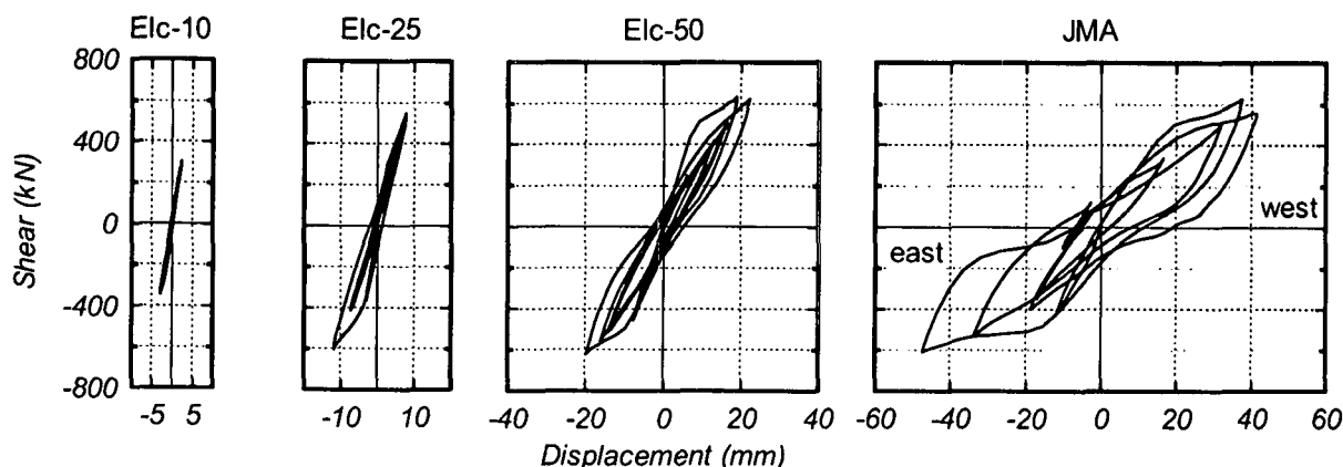
図-6 荷重変形関係(1層部分)
