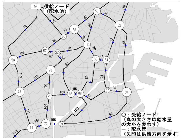
図-3 解析対象の上水道ネットワークの例
