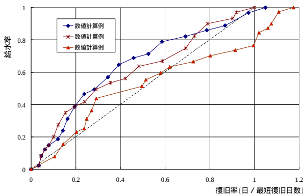
図-8 復旧曲線
