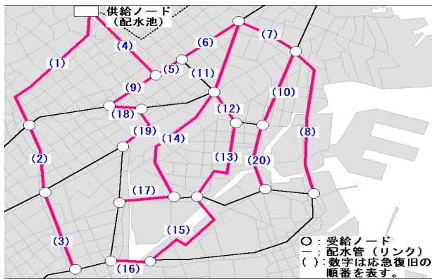
図-7 数値計算例
