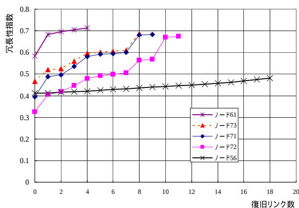
図-5 冗長性指数の値の変化
