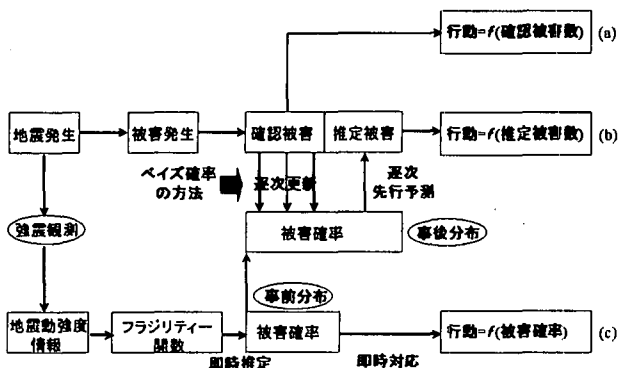
図-1 逐次推定手法と逐次決定過程の概念
