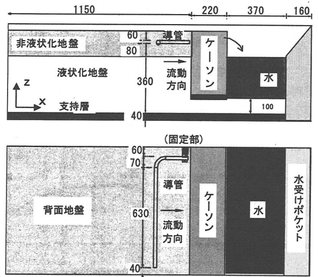
図-5 遠心模型実験の土槽(内曲げ実験時)
