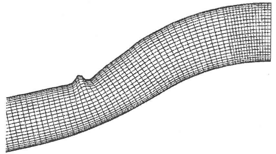
図-4 外曲げによる曲管ならびに直管の変形状況
