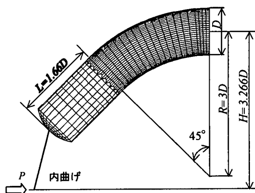
図-1 相似則の確認に用いた有限要素モデル(内曲げ)
