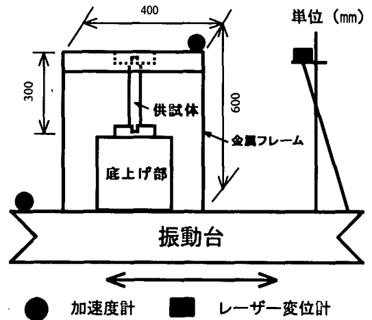
図-2 実験概要図
