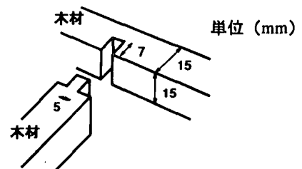
図-3 供試体接合部
