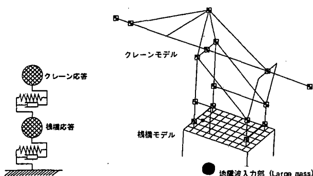
図-5 2 質点 バネモデル概念図
