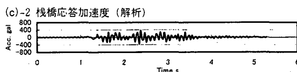
図-9 入力地震波と応答加速度の時刻歴
