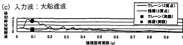
図-8 地震波による応答加速度と橋橋固有周期
