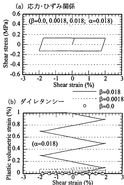
図1 地盤の非線型特性 (Drucker-Prager model)
