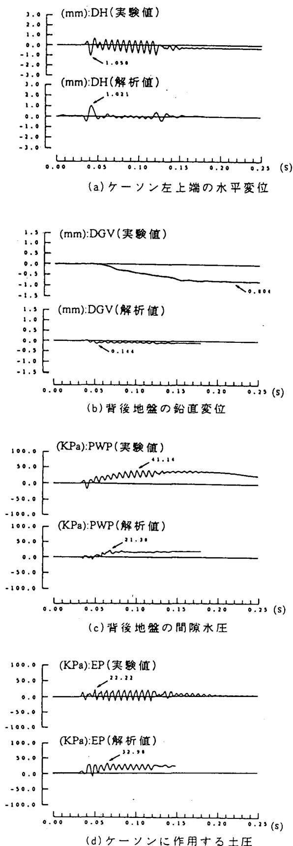
図-3 変位、間隙水圧、土圧の時刻歴の比較
