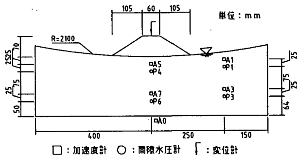
図-1 盛土模型の断面図
