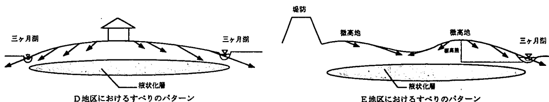
図-6 愛知地区におけるすべりのパターン (断面図)
