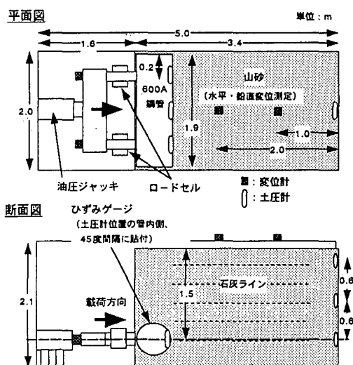
図2 実験装置および計測項目 (口径600Aの場合)
