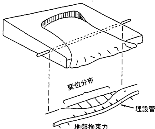
図1 地盤が側方変位した例
