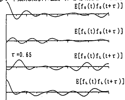
Fig. 8 兵庫県南部地震の場合の相関関数
