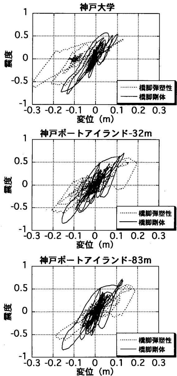
図-6 動的解析における震度-変位関係 (上部構造慣性力作用位置)
