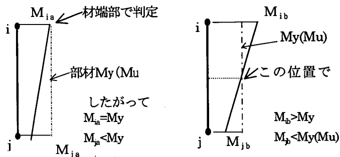
(a) 部材端部での判定 (B社) (b) 部材中央部での判定
