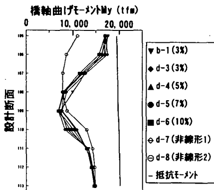
図-9 主桁の剛度及び減衰定別比較 (橋脚応答曲げモーメント)
