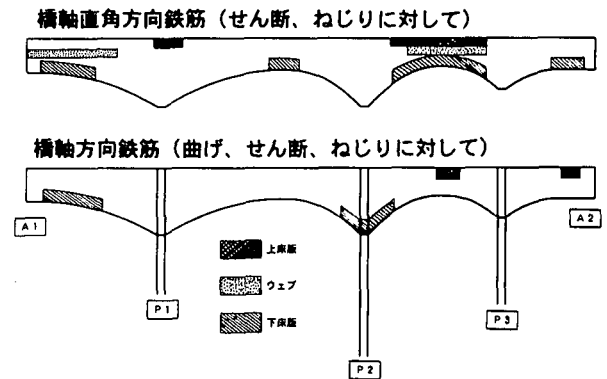
図-10 上部工補強鉄筋配置部位
