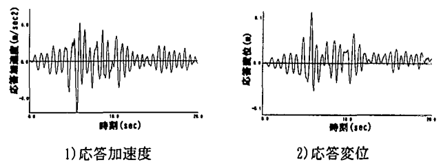
図-3 応答時刻歴
