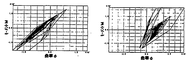
図-4 曲げモーメント～曲率履歴曲線
