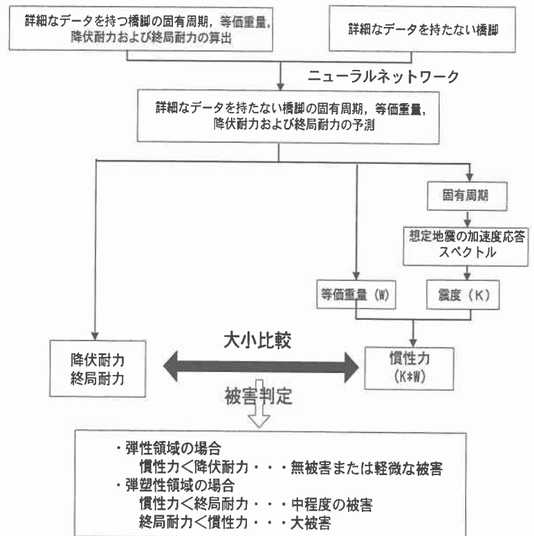
図-5 橋脚の地震被害予測システム
