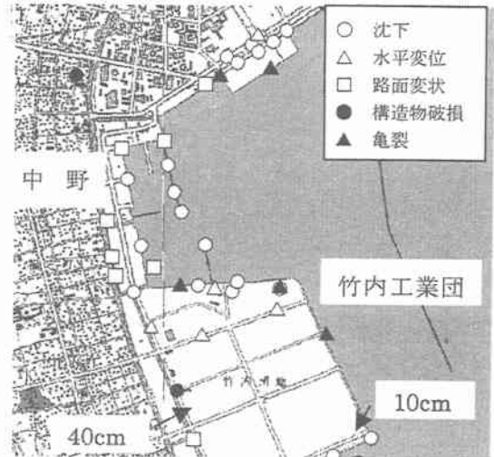
図-4 液状化被害箇所および地盤の沈下量
