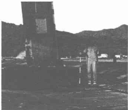
図-2 カニかご護岸の被害
