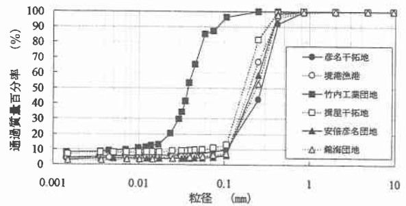
図-6 粒径加積曲線
