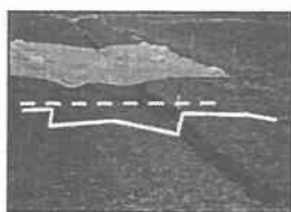
図 7 掬屋干拓地被災状況写真
