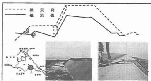
図 10 飯梨川河口付近左岸被災状況
