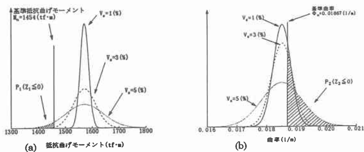
図-7 コンクリートの変動係数5%のときの確率分布
