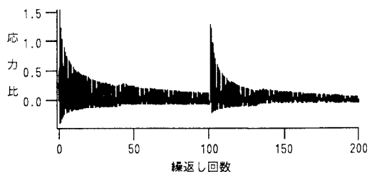
図-4 応力比の時刻歴
