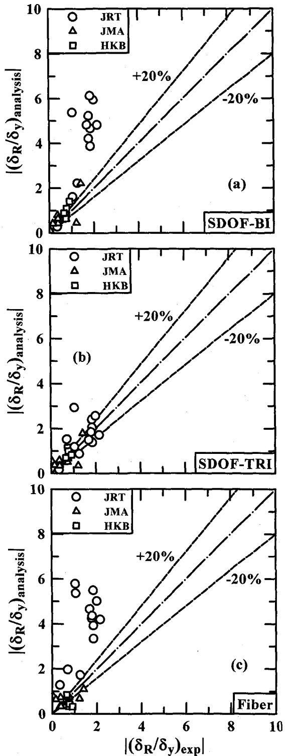
図-9 応答推定手法の精度検証：残留変位
