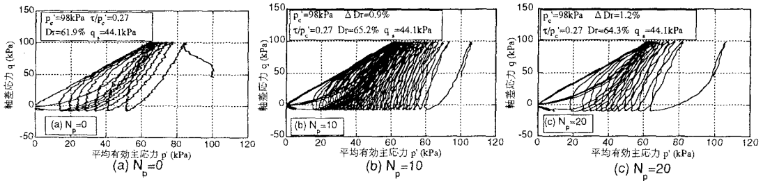
図-2 有効応力径路図
