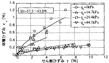
図-7 せん断ひずみ \gamma_p と体積ひずみ \epsilon_v の関係
