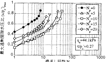
図-3 繰返し回数 N と最大過剰間隙水圧比 (u/p'c)_{max} の関係
