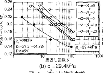
図-4 液状化強度曲線
