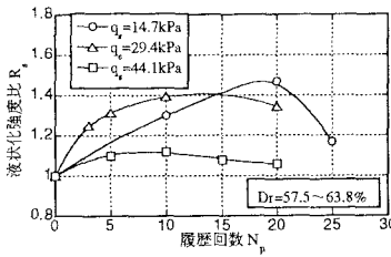
図-5 繰返し履歴回数 N_p と液状化強度比 R_s の関係
