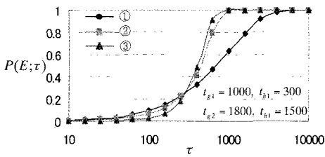
図-4 地震危険度が近い将来で低く、遠い将来で高くなる例
