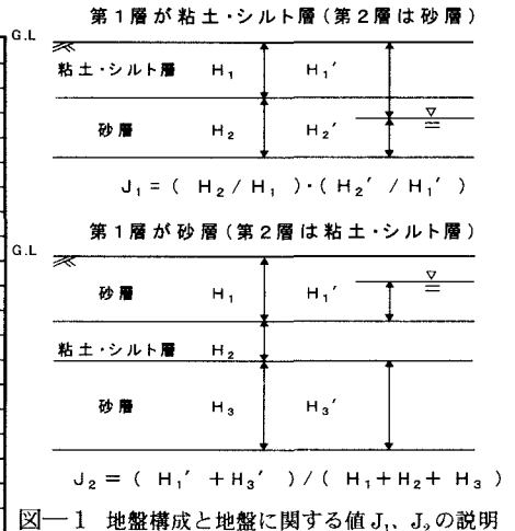
図一 1 地盤構成と地盤に関する値 J_1 、 J_2 の説明
