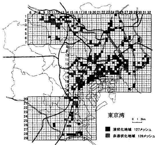
図-2 関東地震時の東京の液状化履歴
