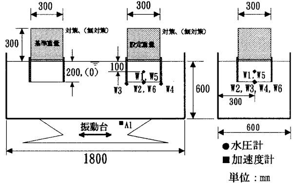
図1 実験概要図
