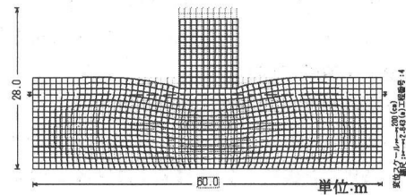
図-2 未改良地盤変形図(変位スケール 1/200)
