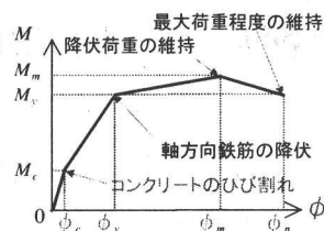
(c) 柱・地中梁部材のモデル化
