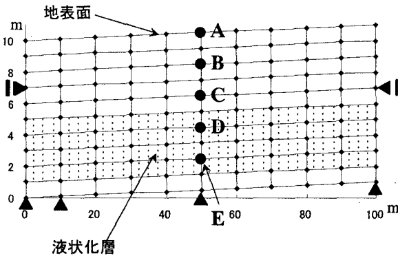
図-1 解析モデル(初期状態)
