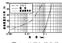
図-2 粒径加積曲線
