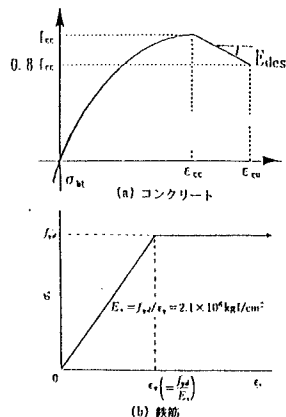
図-2. 応力-ひずみ関係
