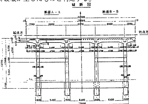
図-1. 構造諸元
