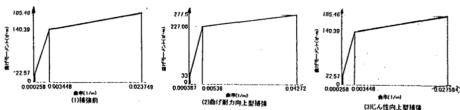
図-3. 曲げモーメント-曲率関係
