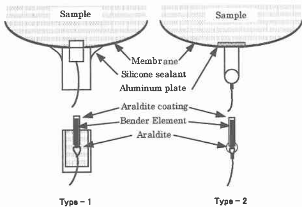
図-2 ベンダーエレメント設置方法
