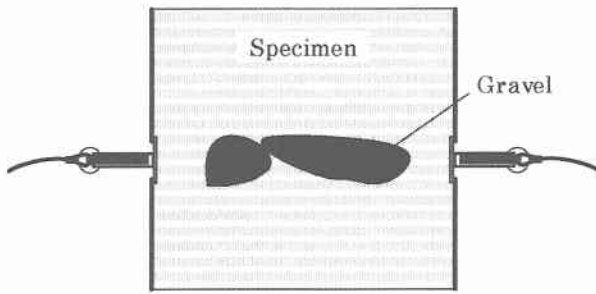
図-7 せん断波の伝播経路に礫を配置
