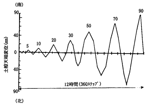
図-5 載荷スケジュール
