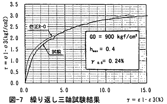
図-7 繰り返し三軸試験結果
