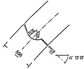
図-2 継ぎ手部構造の例
