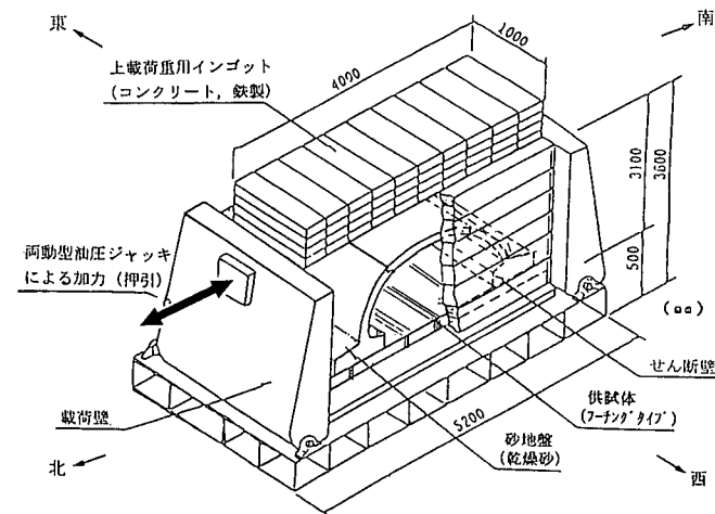
図-4 せん断土槽
