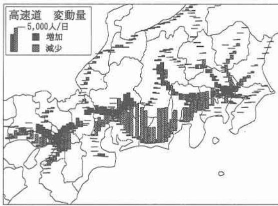
図6 高速道のリンク配分交通量期待変動量
