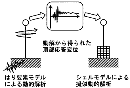
図-7 本解析手法概念図 (擬似的動解)
