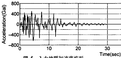
図-6 入力地震加速度波形 (JR 警報地震計観測地震波形 NS 成分)
