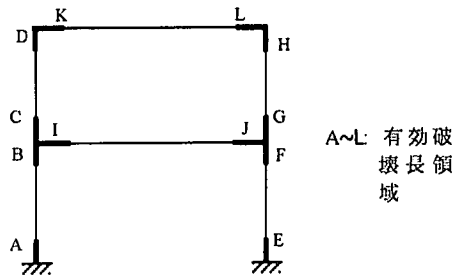
図-6 ひずみの照査領域
