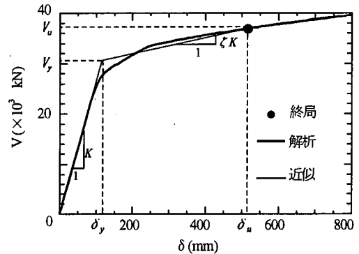
図-4 V-δ曲線の計算結果
