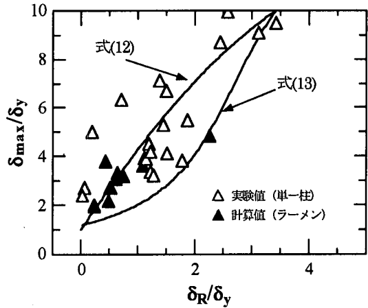
図-9 応答塑性率と残留変位関係
