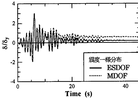
図-5 MDOF と ESDOF の応答変位の比較
