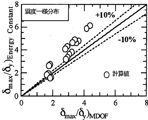
図-8 エネルギー一定則の精度
