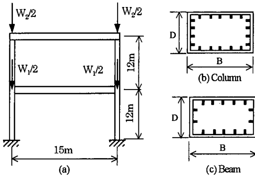
図-3 例題の構造物
