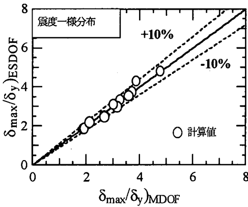
図-7 応答塑性率の比較
