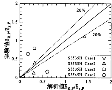
図4 残留変位の比較
