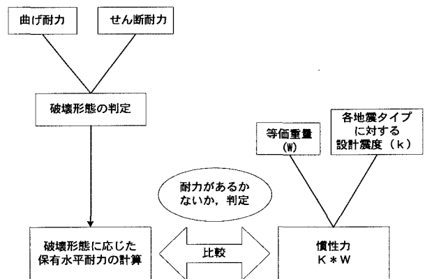
図-2 地震時保有水平耐力法のフローチャート
