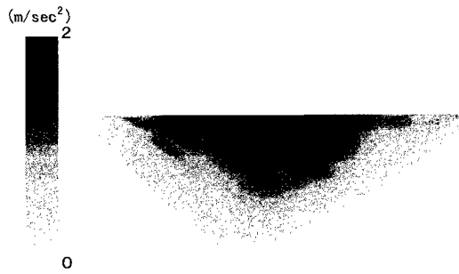
図5 最大加速度分布（三次元解析結果）
