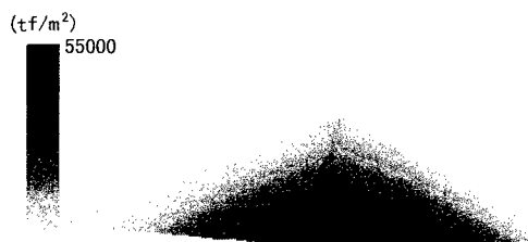
図2 初期物性値（せん断剛性）
