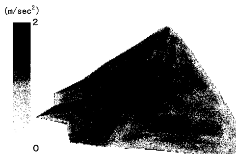
図5 最大加速度分布（三次元解析結果）
