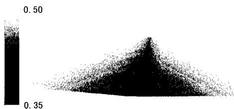
図3 初期物性値（ポアソン比）
