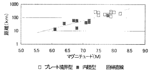
図-3 影響の及んだ最大震央距離とマグニチュードの関係（鉄道被害）
