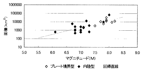
図-4 分布領域の面積とマグニチュードの関係（液状化）
