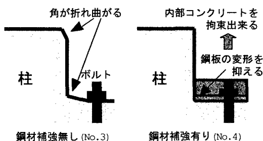
図-3 間仕切りケースの鋼材の効果
