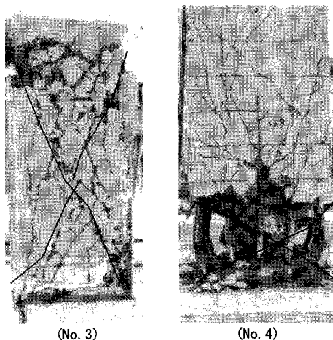
写真-1 鋼板を剥がした後の状況
