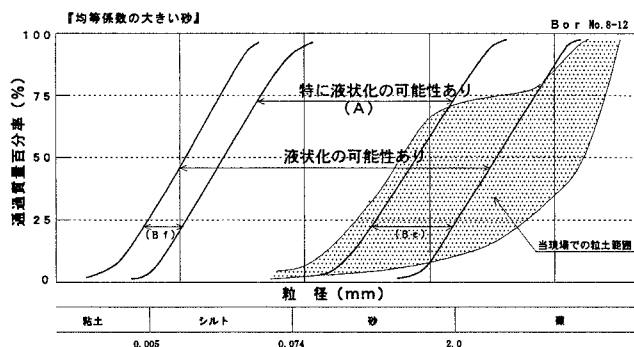
図-3 裏埋土の粒度分布
