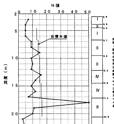
図-4 裏埋土のN値
