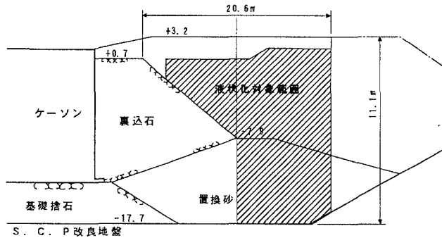
図-2 施工断面図
