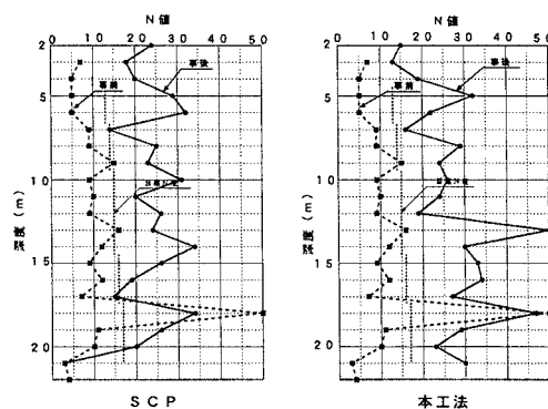
図-6 改良後の杭間N値
