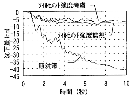
図-4 タンク沈下時刻歴の比較
