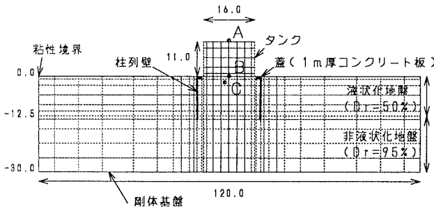
図-1 数値解析モデル
