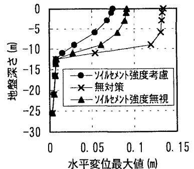
図-6 各解析ケースの水平変位
