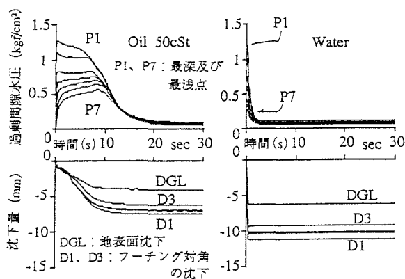
図-4 間隙流体による過剰間隙水圧及び沈下の違い
