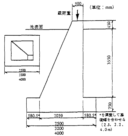
図-1 対象とした送電鉄塔基礎
