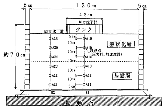
図-1 模型振動実験概要図
