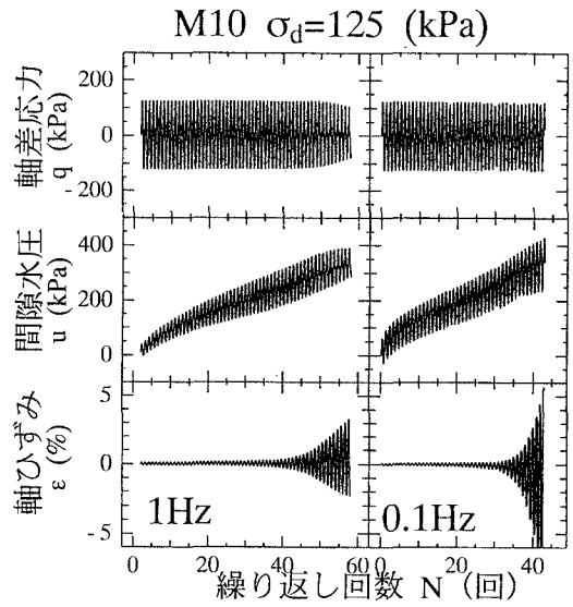
図1 軸差応力, 間隙水圧, 軸歪~繰返し回数の関係
