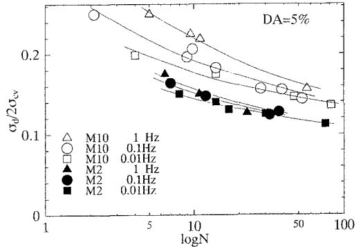
図2 \sigma_d/2\sigma_{cv}' \sim \log N の関係
